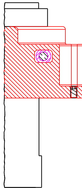
SECTION D-D
